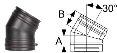
Отвод 30° 7с
