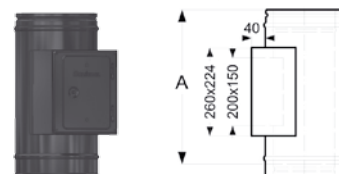
Тройник прочистки для твердого топлива 6с
