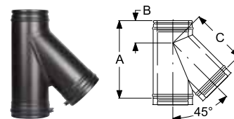
Тройник 45° 6б
