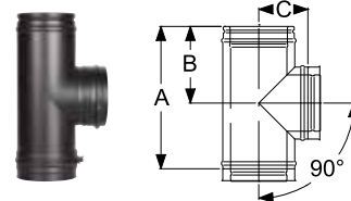
Тройник 90° 6а
