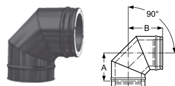
Отвод 90° (Т450 NI) 7а
