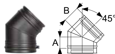
Отвод 45° 7б
